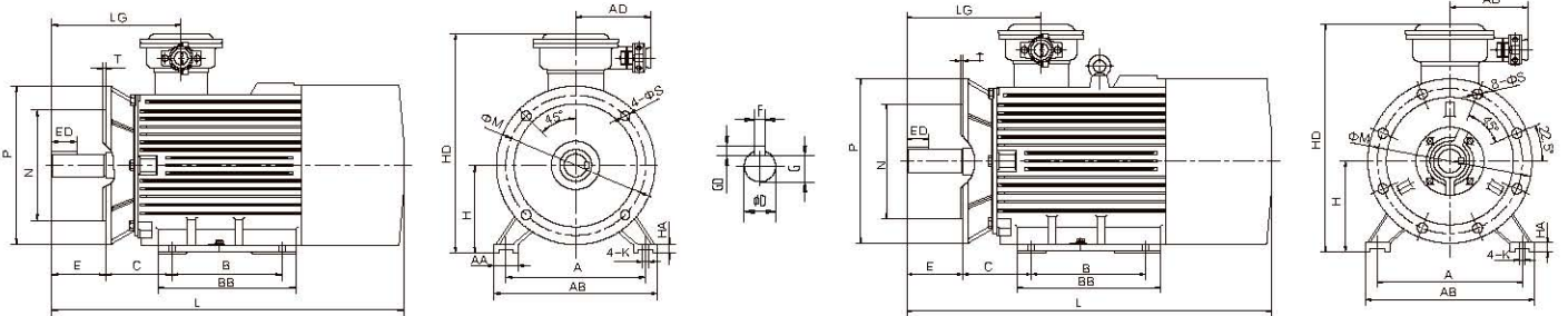
(YBX3-80-200)
