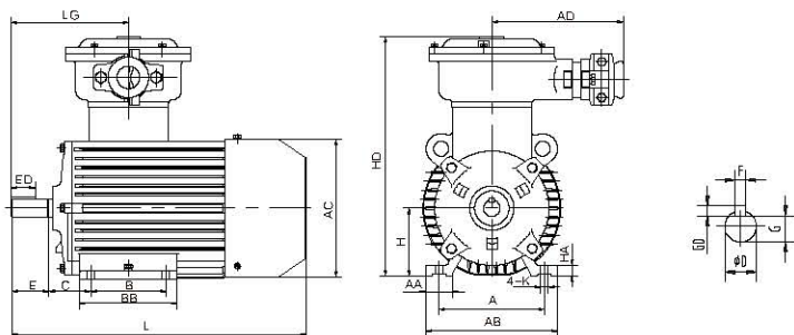
(YBX3-80-160)
