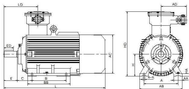
(YBX3-180-355)
